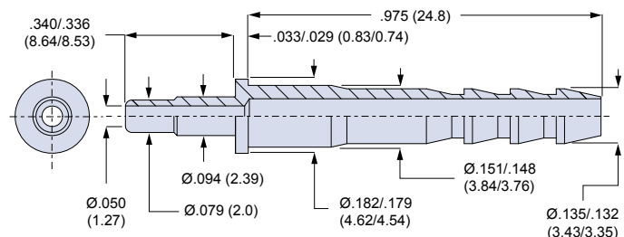
830-003 Pin Contact
