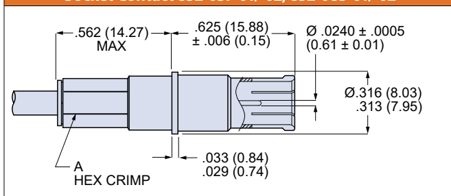
Socket Contact 852-057-01/-02, 852-083-01/-02
