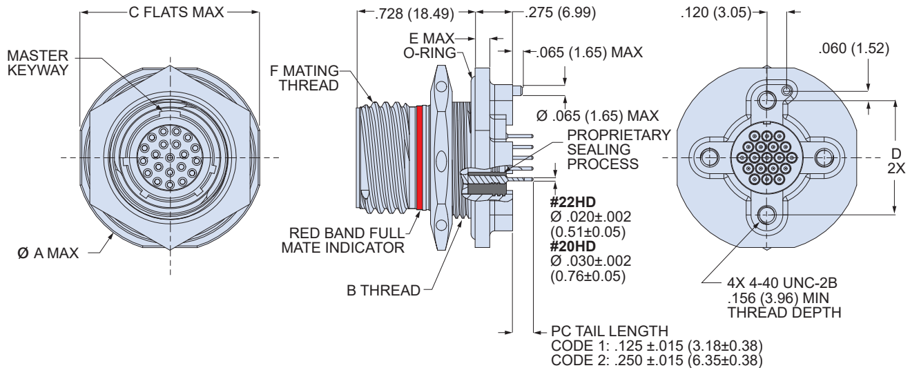
806-028 Receptacle Dimensions
