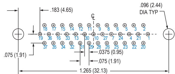
37 SOCKET
