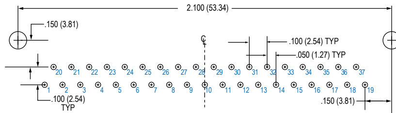
37 SOCKET
