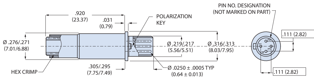
854-001 Pin
