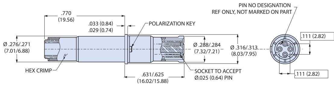
854-002 Socket
