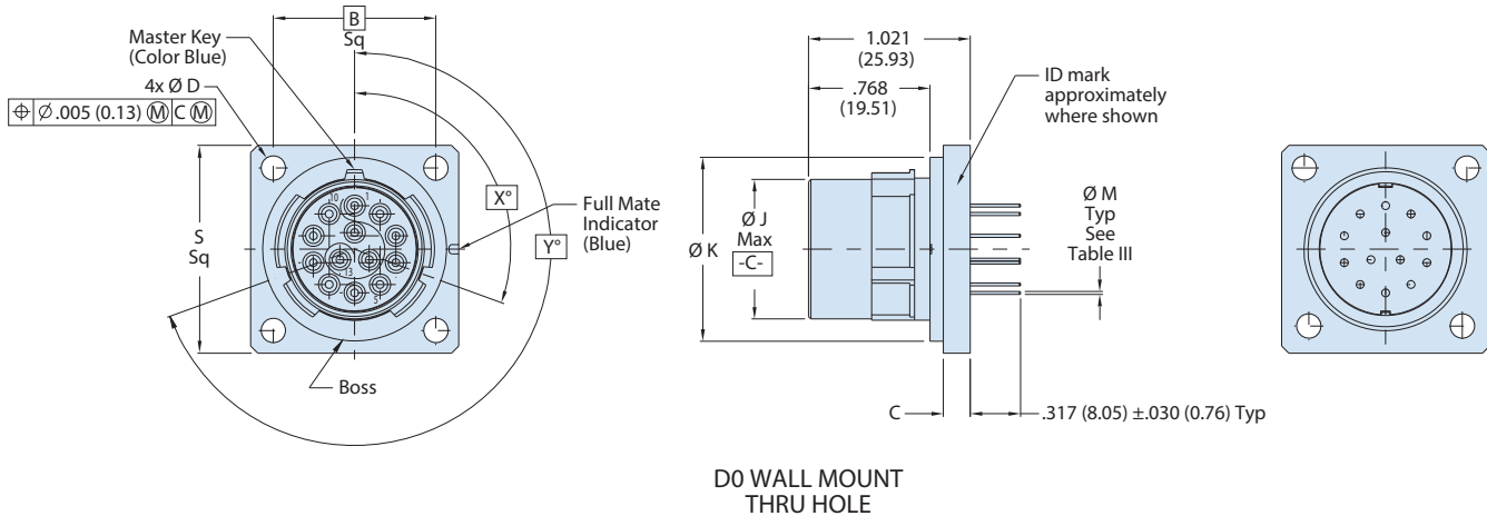
234-207 -D0 WALL MOUNT RECEPTACLE DIMENSIONS
