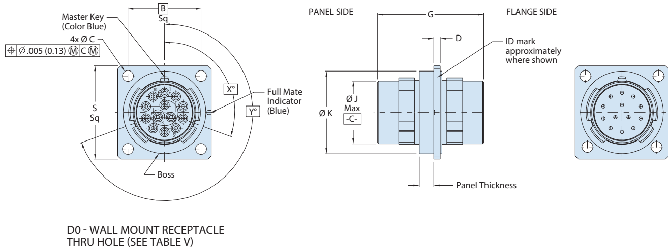
WALL MOUNT RECEPTACLE 234-212 - D0
