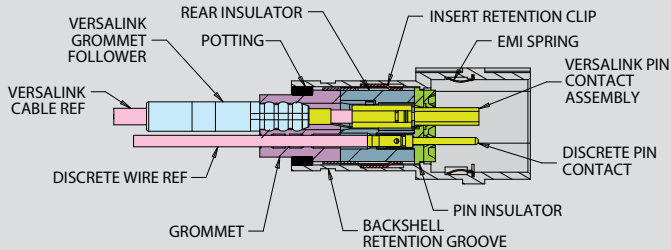
794-002 CABLE RECEPTACLE
